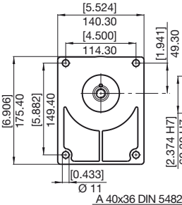
A 40x36 DIN 5482
