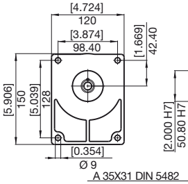
A 35X31 DIN 5482
